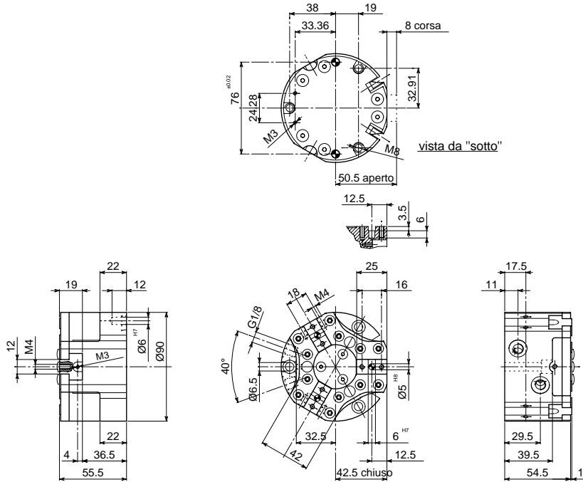
• Disegno QPG 309 • Drawing QPG 309 • Zeichnung QPG 309 • Dessin QPG 309
